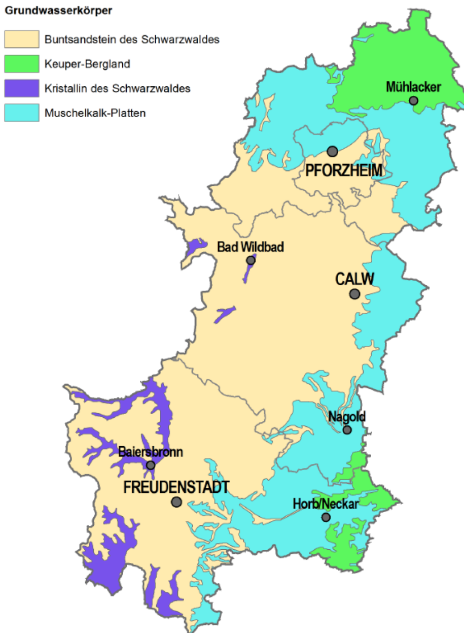
Abbildung 9: Grundwasserkörper (RVNSW 2018).
